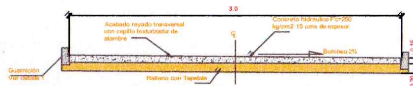
SECCION TRANSVERSAL DE PAVIMENTO
