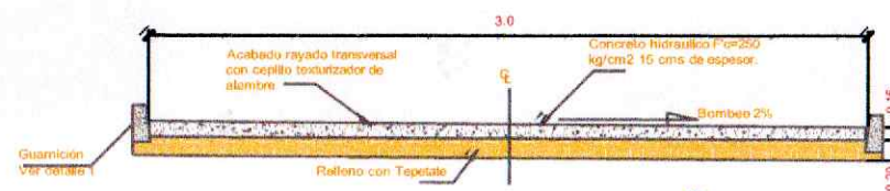
SECCION TRANSVERSAL DE PAVIMENTO
