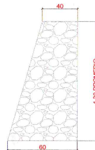
DETALLE 3 MURO DE MAMPOSTERIA
