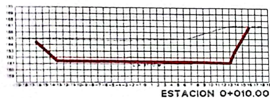
ESTACION 0+010.00
