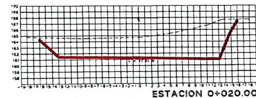
ESTACION 0+020.00
