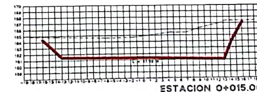
ESTACION 0+015.00
